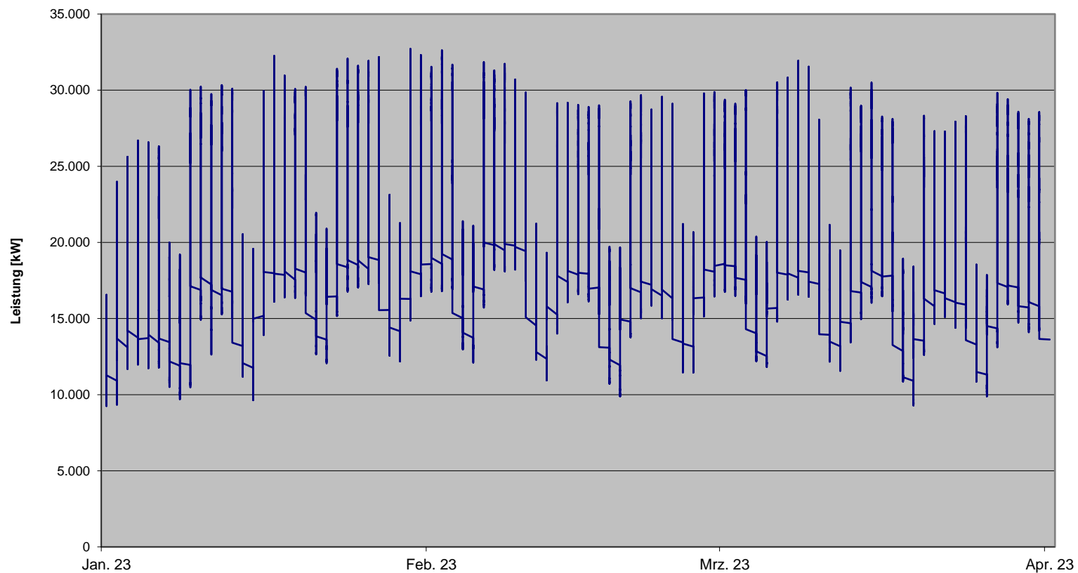
Jahreshöchstlast aller Spannungsebenen - Geschäftsjahr 2023 (1. Quartal)
